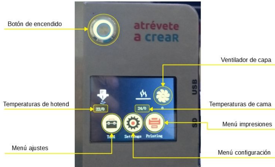
Símbolos de pantalla principal LCD y botón de encendido.
