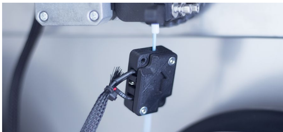
Sensor de filamento en posición usual, cerca del extrusor
