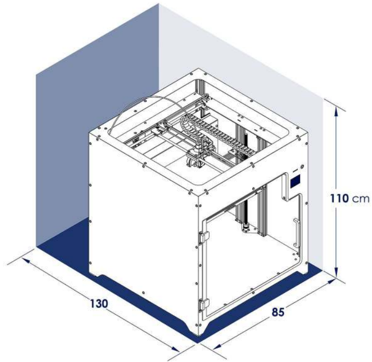
Ilustración del espacio mínimo requerido para instalar la máquina.
