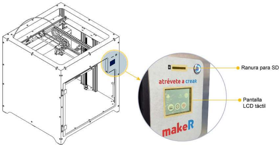
Ubicación de la pantalla LCD y de ranura de inserción de tarjeta SD
