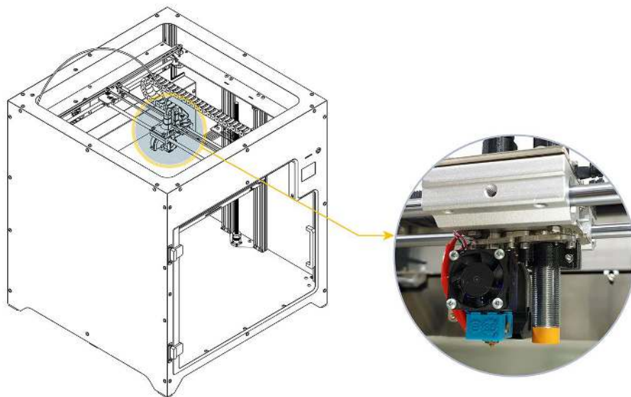
Ubicación y detalle del Hotend de la impresora 3D
