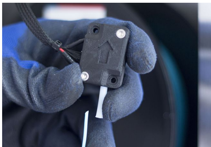
Sensor de filamento con la flecha indicadora de dirección
